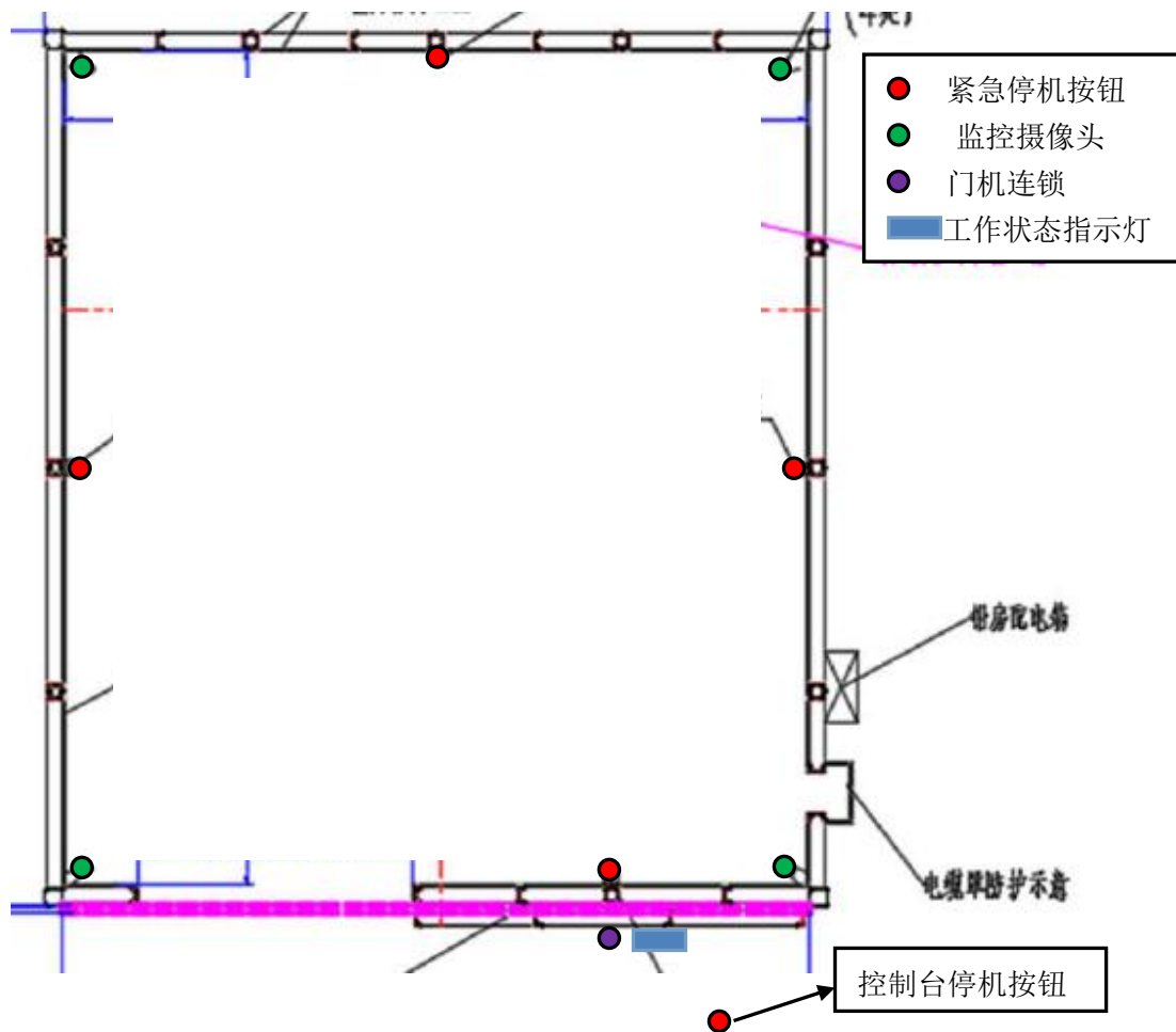
图 10-3 安全裝置所在位置示图
